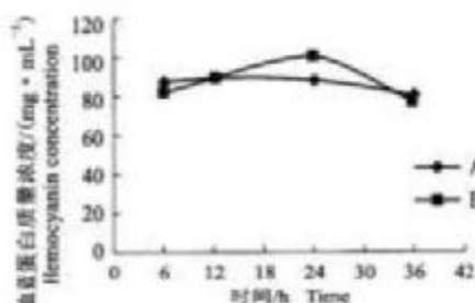
图1 南美白对虾感染副溶血弧菌后血清血蓝蛋白的浓度变化
