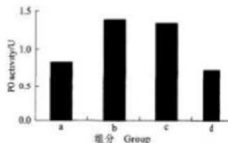
图5 南美白对虾血清蛋白重组蛋白对其血清酚氧化酶活力的影响
