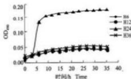
图2 南美白对虾感染副溶血弧菌后血清酚氧化酶活力动力曲线
