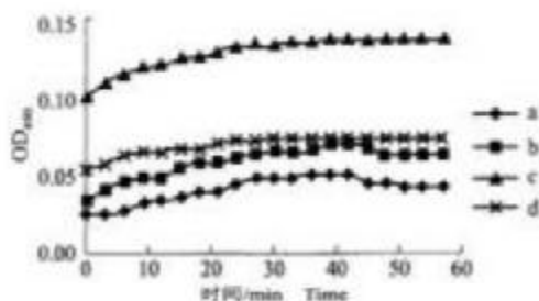
图4 南美白对虾血清蛋白重组蛋白对其血清酚氧化酶活力影响的动力曲线
