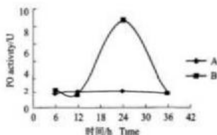
图3 南美白对虾感染副溶血弧菌后血清中酚氧化酶活力的变化
