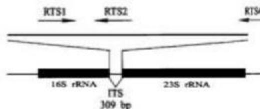
图2 真核生物核糖体操纵子及用于鲑鱼立克次氏体 ITS 区域 PCR 扩增的引物对 RTS1-RTS2、RTS1-RTS4 位置图 [28]
