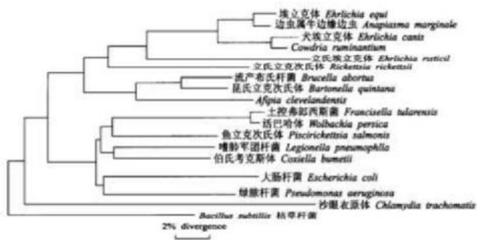
图 1 鲑鱼立克次氏体与经选择的立克次氏体和细菌系统发生学关系图 [1]
