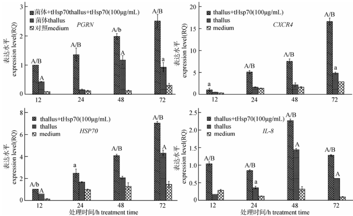
图 6 tHSP70 对腹腔巨噬细胞免疫相关基因表达影响的时间效应
