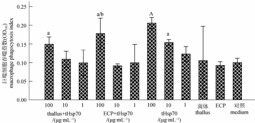
图 4 tHsp70 对体外培养罗非鱼腹腔巨噬细胞吞噬活性的影响
